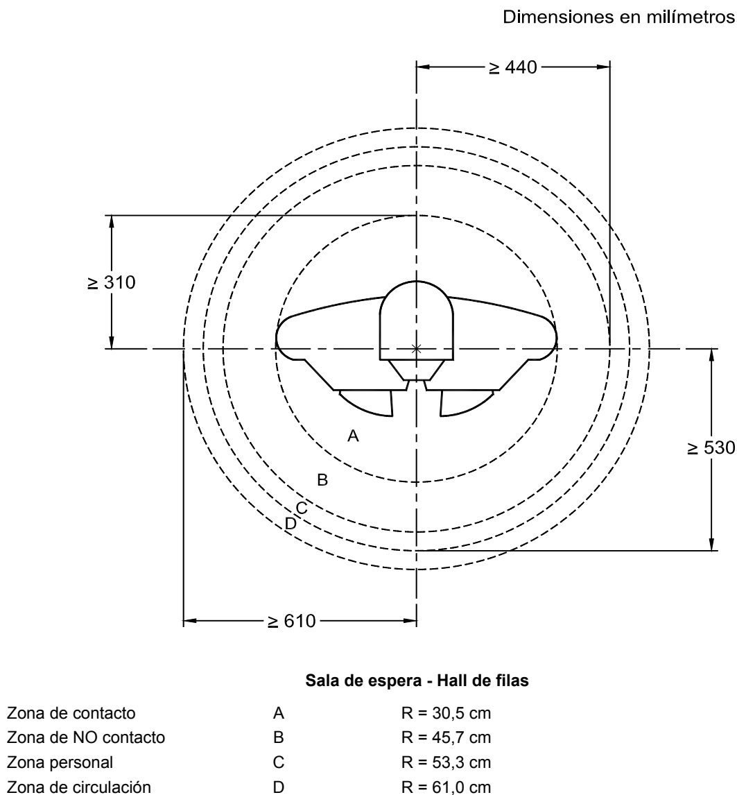
Figura 33 Espacio de circulación de una persona
