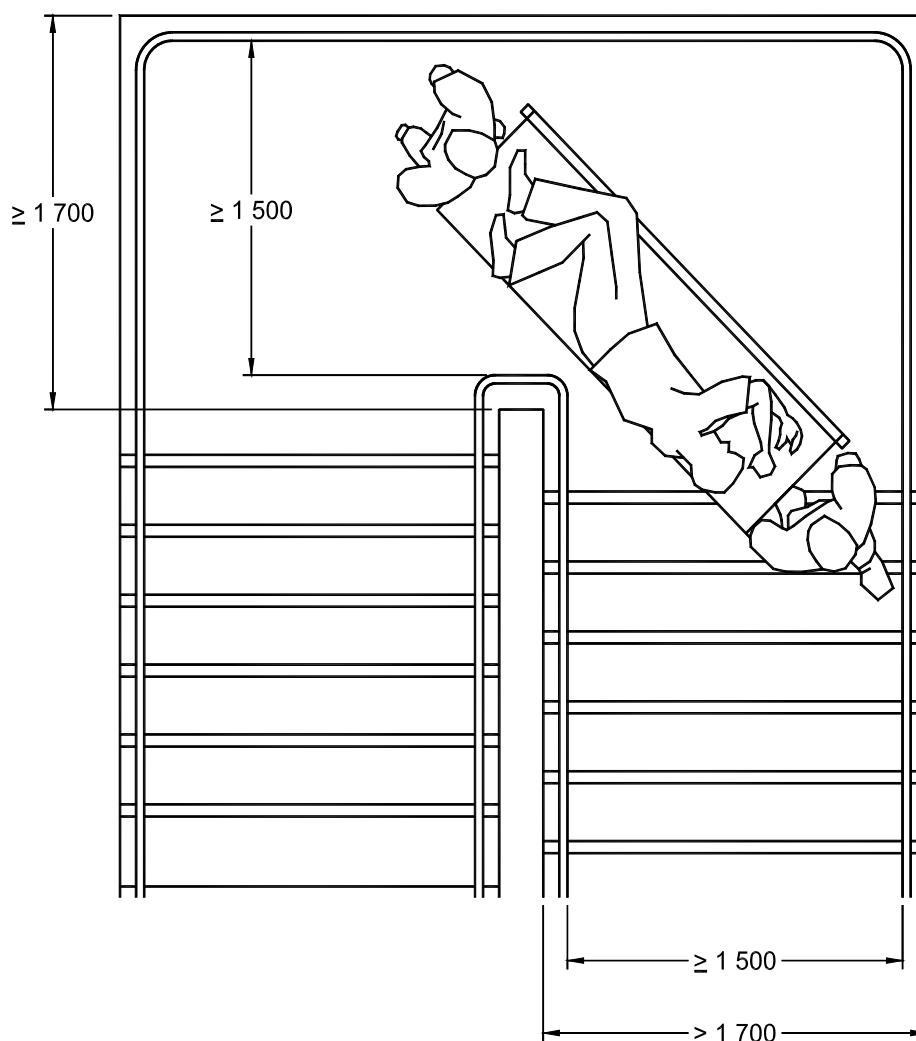
Figura 15. Ejemplo de escalera y descanso de 180° para acceso de emergencia
