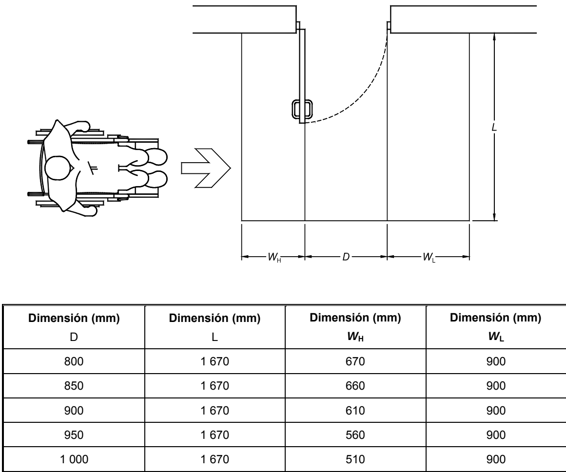
Figura B.5. Espacios de circulación en entradas con puertas de batiente - bisagra lateral: la puerta abre hacia el usuario
