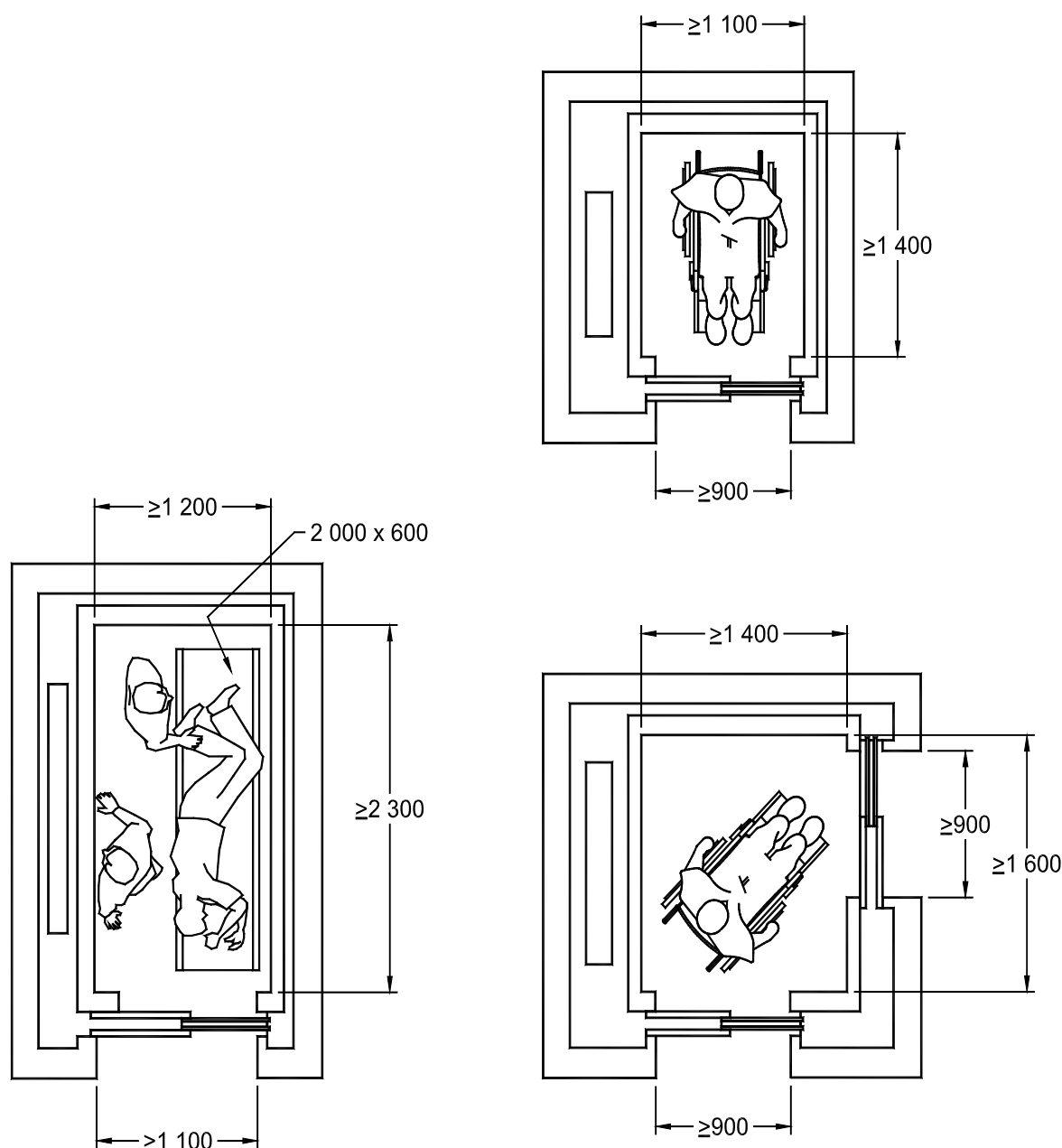
Figura 19. Ejemplos de ascensores que permiten acomodar una persona en silla de ruedas, una persona en una camilla y una persona que realice un giro de 90° entre dos puertas de ascensor adyacentes.
