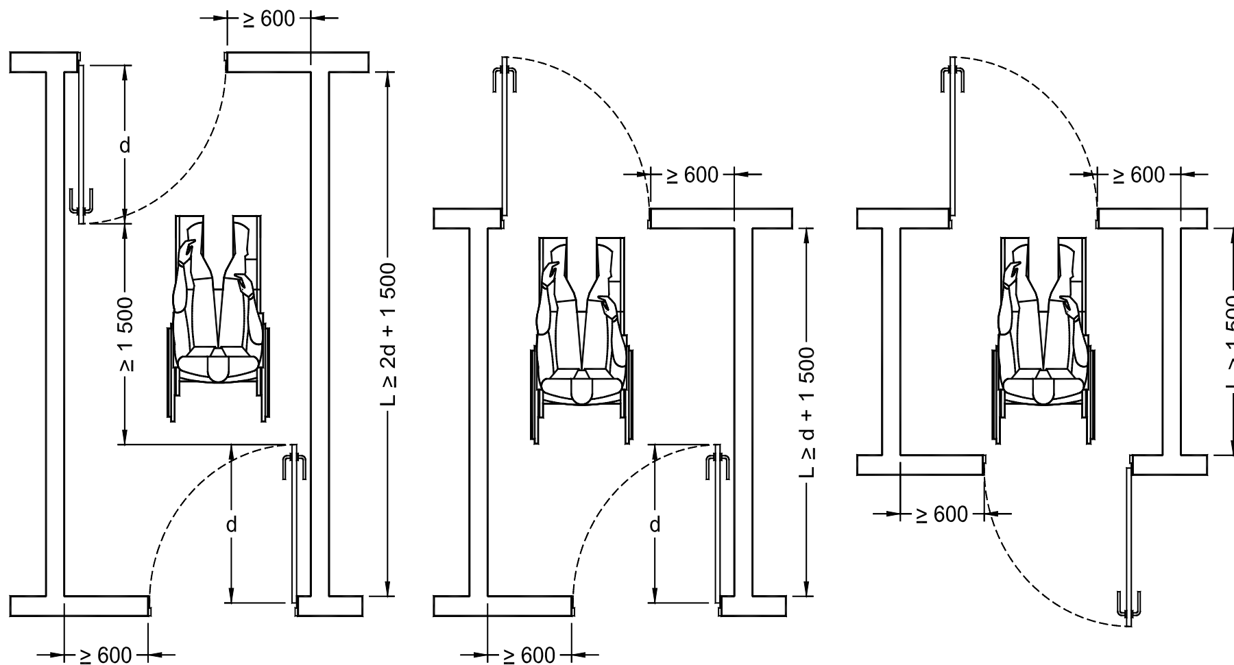
Figura 31. Dimensiones mínimas de los vestíbulos con puerta batiente de una sola hoja
