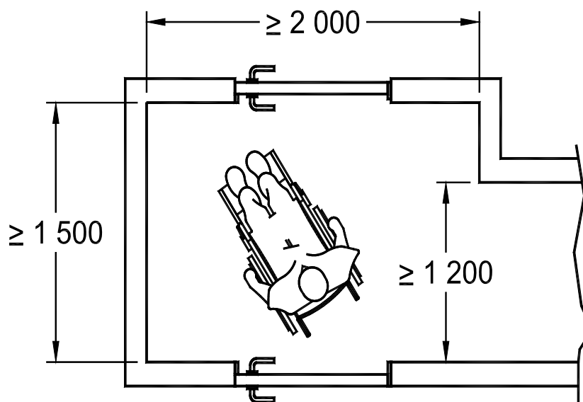
Figura 11. Espacio requerido para un giro de 180° en un corredor
